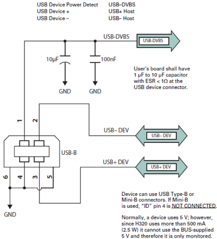
图 2-4 USB device设计参考电路
