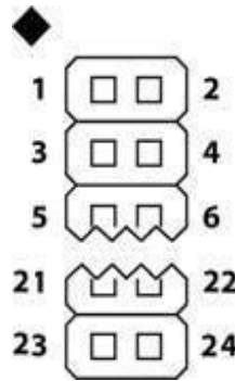
图 2-2 H328 24-pin针脚表
